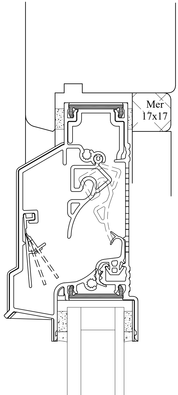
BUVA Slidestream 12 rooster Glasgoot 26, 30 en 34mm HR++ Dubbelglas
